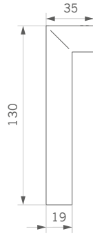
Toi raamkruk L-model haaks ø19mm
