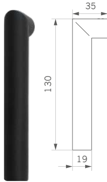
Toi raamkruk L-model haaks ø19mm
